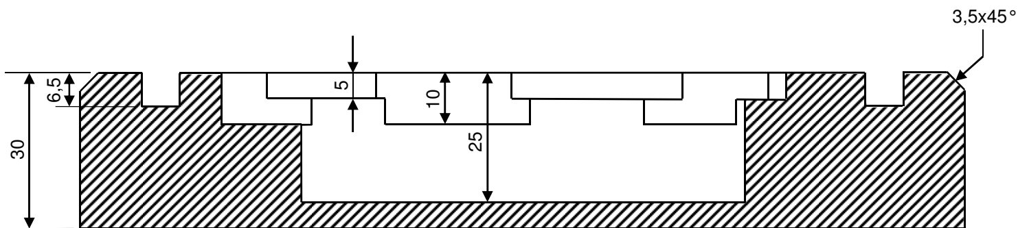
section A-A
